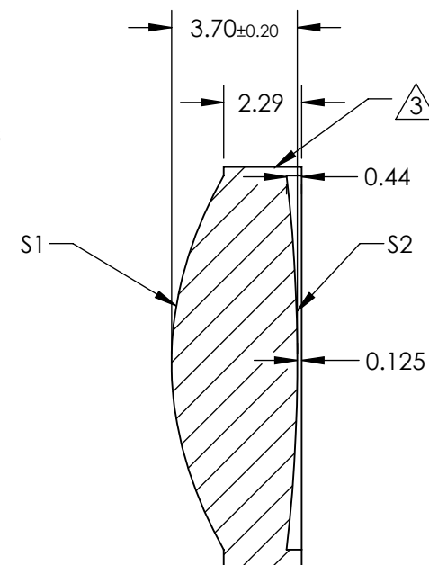
SECTION A-A
