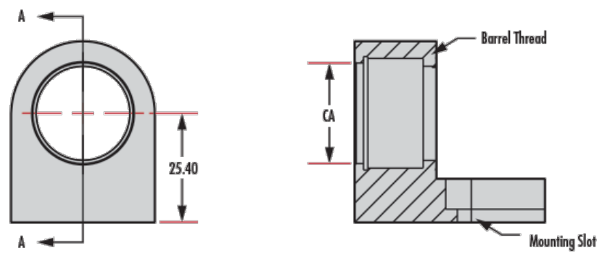
L-Slot Type (#36-410 & #36-416)
