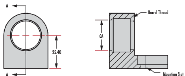
L-Slot Type (#36-410 & #36-416)
