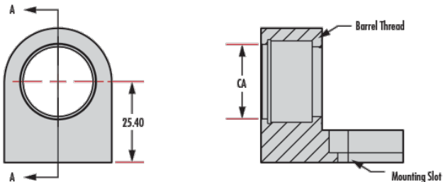
L-Slot Type (#36-410 & #36-416)
